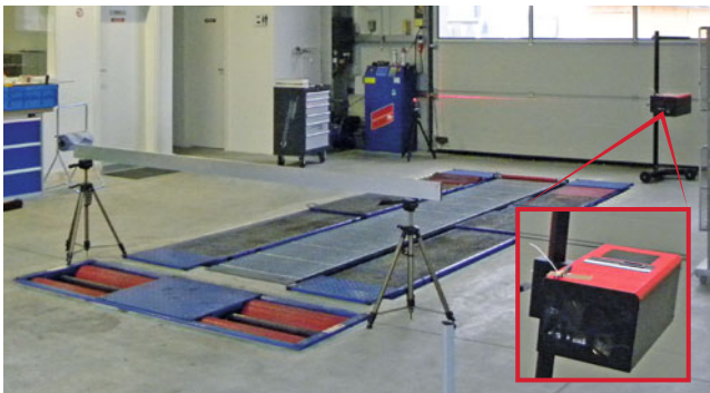
Bild 1: Estrichboden mit Messaufbau, Linienlaser für Bezugsebene, Punktlaser auf Optikkasten, Richtschieit als Projektionsebene (Quelle: GTÜ)
