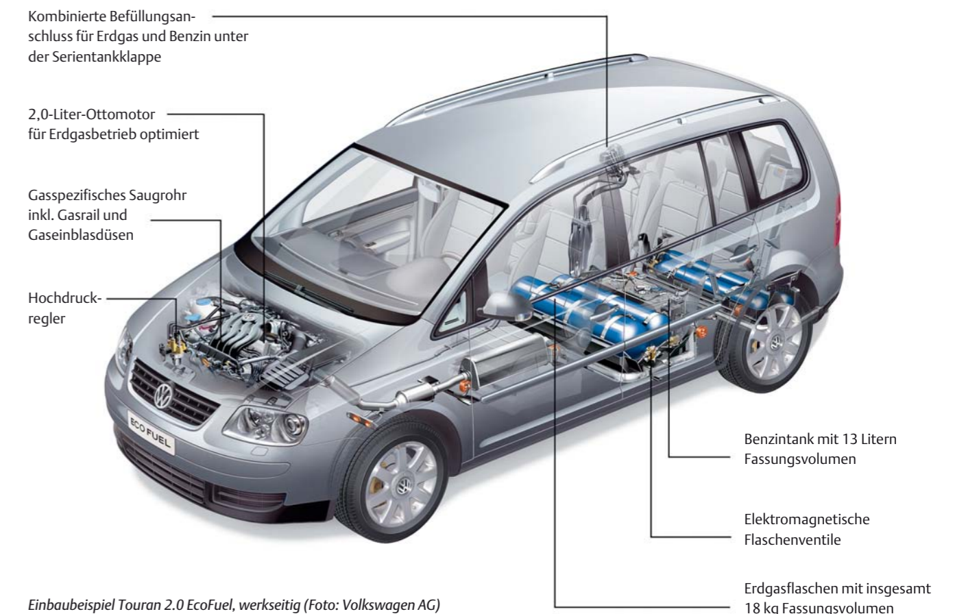
Einbaubeispiel Touran 2.0 EcoFuel, werkseitig (Foto: Volkswagen AG)
